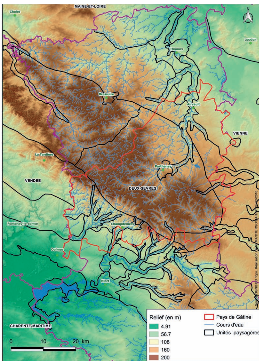
Carte du relief du Pays de Gâtine
