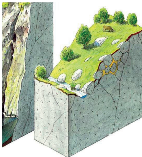
Bloc diagramme de la formation de « chirons » (Charte paysagère)
